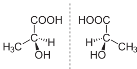
Abbildung 49 Milchsäure (S) und (R) 24
