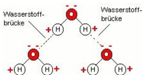
Abbildung 11 Wasserstoffbrückenbindung
