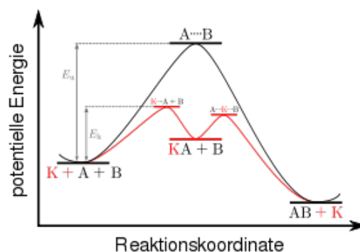
Abbildung 19 Katalyse einer Reaktion, es ist gut ersichtlich wie 2 Übergangszustände gebildet werden
