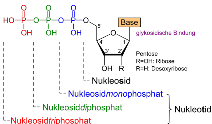
Abbildung 59 Schematische Darstellung eines Nucleotids 31
