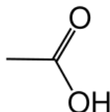
Abbildung 15 Skelettformel von Essigsäure
