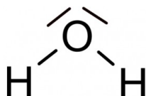
Abbildung 14 Valenzstrichformel für Wasser
