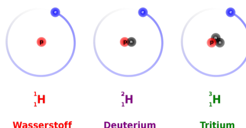
Abbildung 20 Wasserstoffisotope 13
