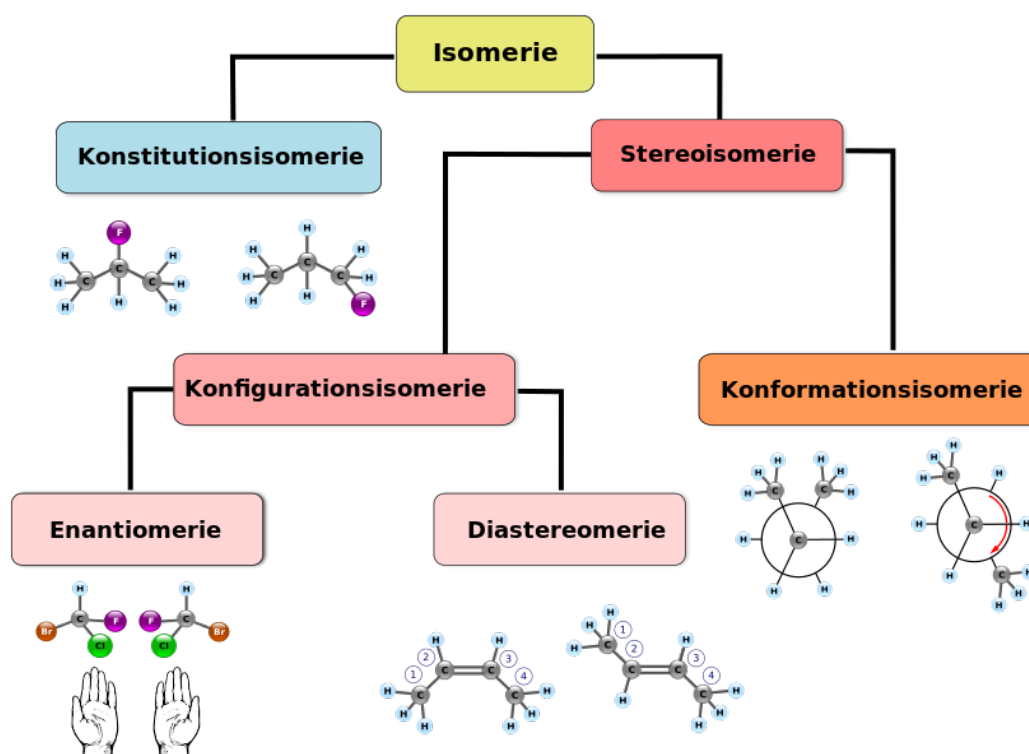
Abbildung 47 Übersicht über die wichtigsten Arten der Isomerie 23
