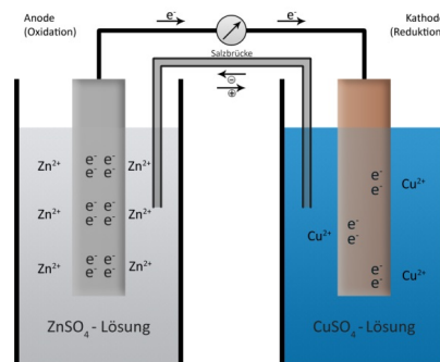
Abbildung 22 Daniell-Element 15
