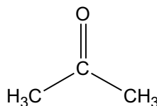
Abbildung 41 Propan-2-on (Aceton)
