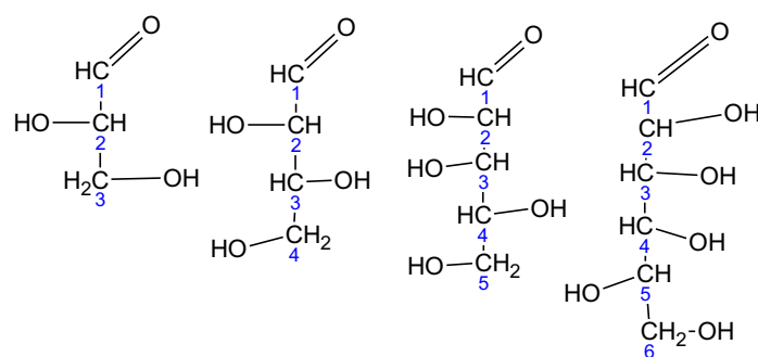
Abbildung 51 Darstellung einer Triose, Tetrose, Pentose und einer Hexose
