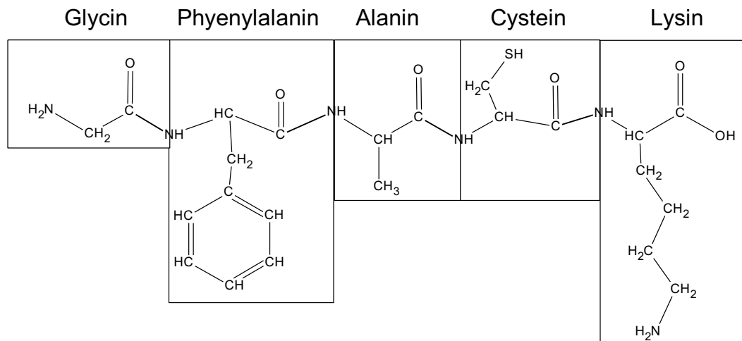
Abbildung 58 Darstellung einer Primärstruktur
