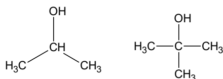
Abbildung 37 Links, Propan-2-ol ein sekundärer Alkohol, Rechts, 2-Methyl-propan-2-ol ein tertiärer Alkohol
