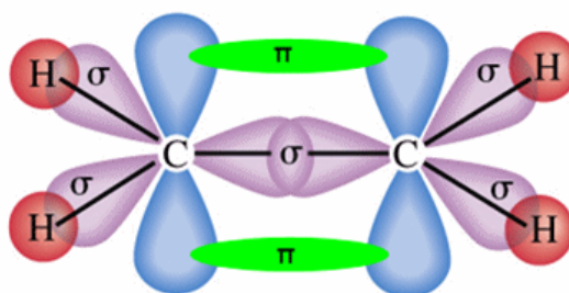
Abbildung 27 Bindungen im Ethenmolekül 20
