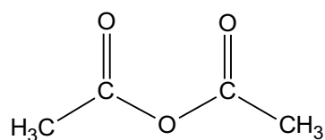
Abbildung 46 Essigsäureanhydrid
