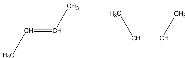
Abbildung 50 trans-But-2-en
