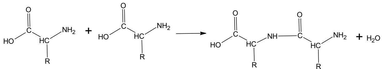
Abbildung 57 Amidbildung unter Wasserabspaltung (Kondensation)
