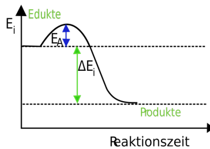
Abbildung 18 E_A die Aktivierungsenergie, E_i die frei Reaktionsenergie, bezieht sich auf eine Exotherme Reaktion 12
