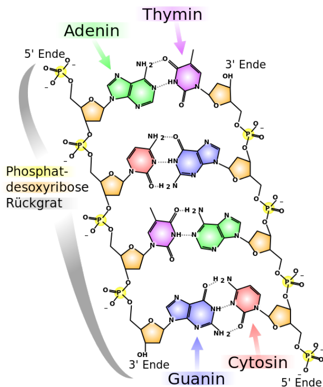
Abbildung 60 Schematischer Ausschnitt aus der DNA 32
