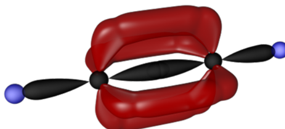
Abbildung 28 Ethinmolekül mit 2 pi-Bindungen und einer sigma-Bindung 21
