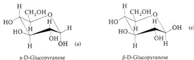
Abbildung 16 Konformationsformeln 10
