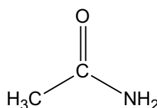
Abbildung 43 Ethansäureamid
