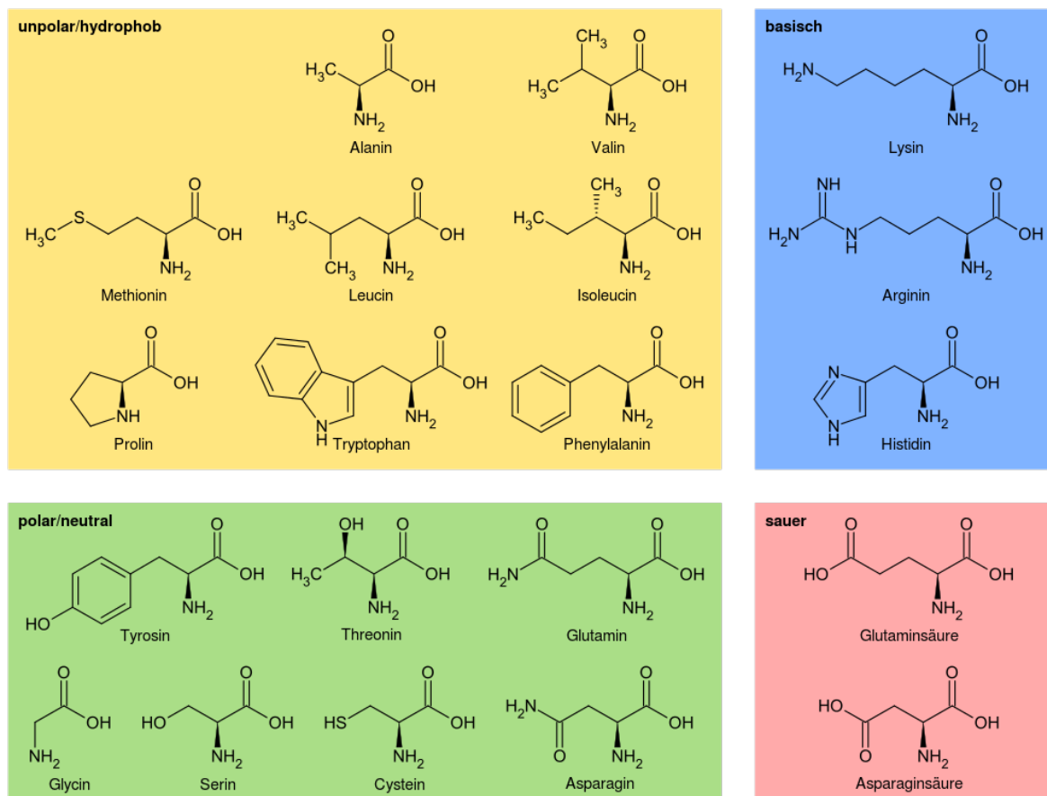
Abbildung 56 20 Proteinogene Aminosäuren 30
