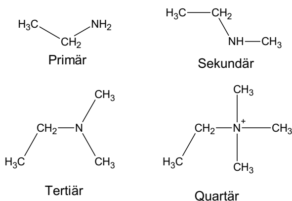
Abbildung 40 Primäres, Sekundäres, Tertiäres und Quartäres Amin
