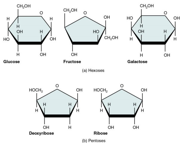
Abbildung 53 Monosaccharide 25
