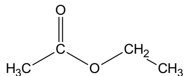
Abbildung 45 Ethansäureester
