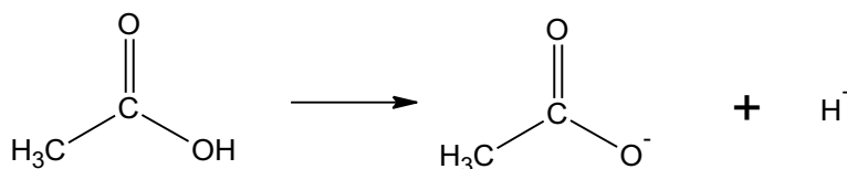
Abbildung 42 Ethansäure und ihre protonendonation (Abgabe eines H + -Ions)
