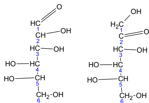
Abbildung 52 Aldose und Ketose
