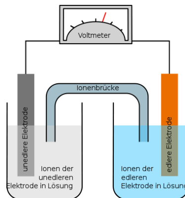
Abbildung 23 Allgemeiner Aufbau einer Galvanischen Zelle 16
