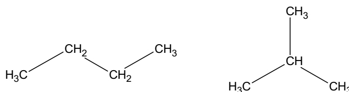
Abbildung 31 n-Butan und Isobutan
