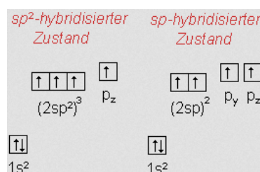
Abbildung 25 sp 2 - und sp-Hybridisierung 18
