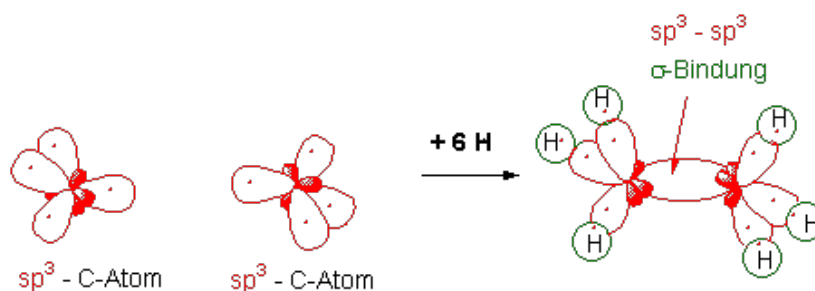
Abbildung 26 Darstellung eines Ethanmoleküls 19
