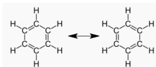
Abbildung 29 Abwechselnde Doppelbindungen
