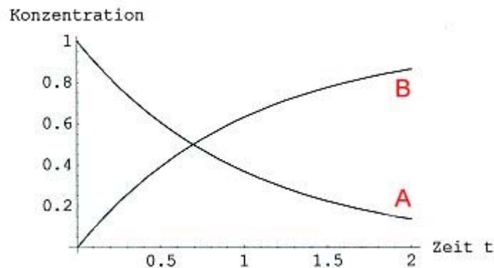
Abbildung 17 Konzentrationsänderung von Reaktanten A und B in Abhängigkeit der Zeit 11
