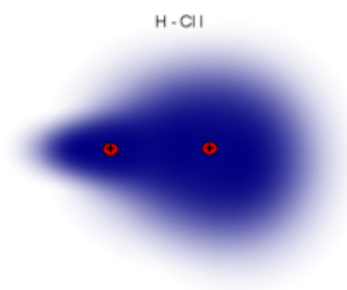
Abbildung 6 Überlagerte Aufenthaltswahrscheinlichkeiten/Orbitale beim HCl Molekül 6
