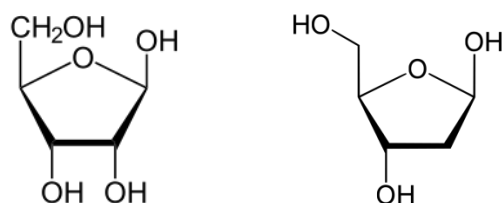
Abbildung 62 Ribose 34 und Desoxyribose 35
