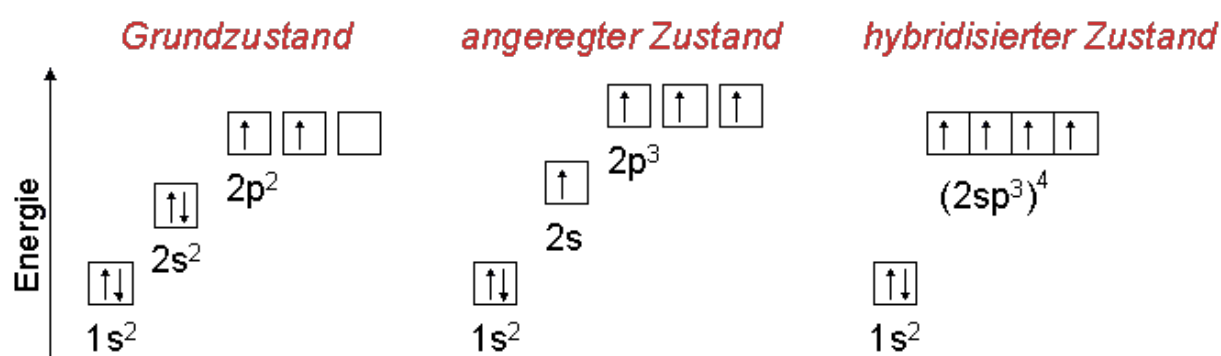
Abbildung 24 Darstellung der Elektronenkonfiguration des Kohlenstoffs 17
