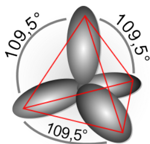
Abbildung 7 sp^3 -Hybridorbital 7
